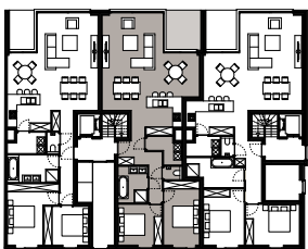
plan gelijkvloers
