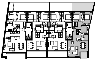
plan eerste verdieping
